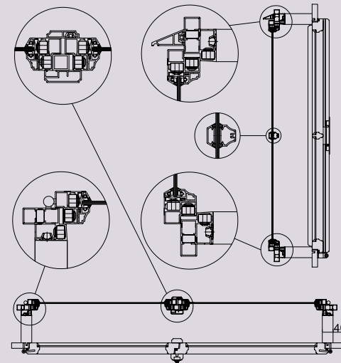
Schnitt Außenöffnend
